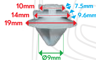
AGRAFE GRILLE BAIE AVENT
