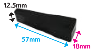
VB4000501 CALE CAOUTCHOUC Coccinelle (11-), Scirocco III (08-)
