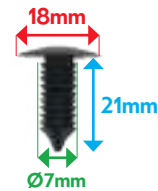
VB4000712 AGRAFE TOLE AUVENT
