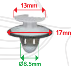
VB20305 AGRAFE PANNEAU DE PORTE R11, R18, R5, R9
