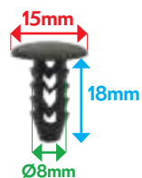
VB4000720 AGRAFE TOLE AUVENT
