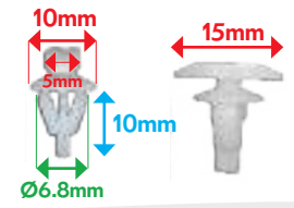
VB4000716 AGRAFE TOLE AUVENT
