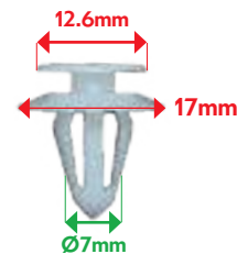
VB56305 AGRAFE PANNEAU DE PORTE Astra, Corsa, Tigra, Vectra, Zafira
