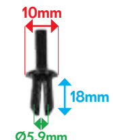
VB4000721 AGRAFE TOLE AUVENT
