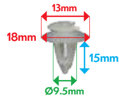
VB4000711 AGRAFE TOLE AUVENT
