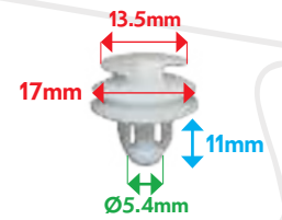
VB4000718 AGRAFE CACHE MOTEUR
