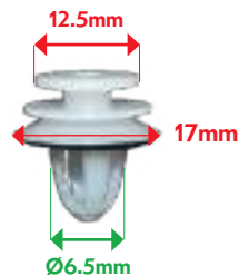
VB3101007 CLIP PB BLANC R56 (07-), R57 (09-), cabrio et Clubman R55 (08-), R50, R53 et cabrio R52 (01-06)
