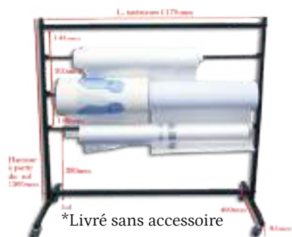
*Livré sans accessoire DÉVIDOIR SUR ROULETTES TRIPLE SUPPORTS
