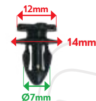
VB82327 CLIP LATÉRAL Fabia II (07-)
