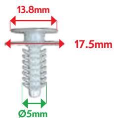
VB59405 AGRAFE PANNEAU DE PORTE Kappa, Nuova, Delta, Y, Ypsilon
