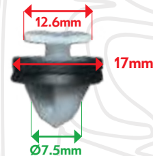
VB19105 AGRAFE PANNEAU DE PORTE Ulysse et Scudo
