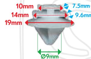
VB17105 AGRAFE GRILLE BAIE AUVENT Nouvelle Clio, Megane III
