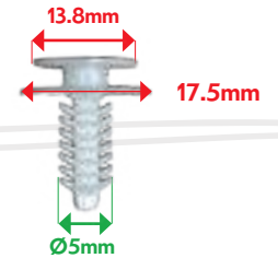
VB59405 AGRAFE PANNEAU DE PORTE Brava, Bravo, Doblo, Marea, Punto (99-03), Palio, Siena, Stilo, Strada, Tempra, Tipo, Panda <03, Punto 03...
