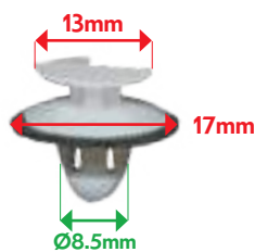
VB20305 AGRAFE PANNEAU PORTE AX, BX, GS et LNA
