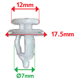
VB72205 AGRAFE PANNEAU DE PORTE Partner
