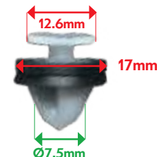
VB19105 AGRAFE PANNEAU DE PORTE Clio II, Clio III, Megane, Kangoo, Kangoo II
