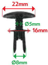
VB3106003 AGRAFE CACHE MOTEUR ESSUIE GLACE Golf III (91-97)
