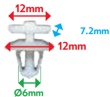
VB12029 AGRAFE BAIE AUVENT Berlingo et Partner
