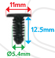
VB4000715 AGRAFE TOLE AUVENT
