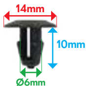
VB4000722 AGRAFE TOLE AUVENT
