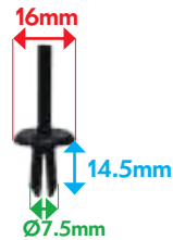
VB4000708 AGRAFE CACHE MOTEUR
