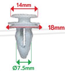
VB32305 AGRAFE PANNEAU DE PORTE Logan
