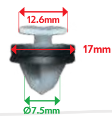
AGRAFE PANNEAU PORTE
