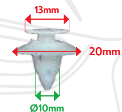
VB72155 AGRAFE PANNEAU DE PORTE KA
