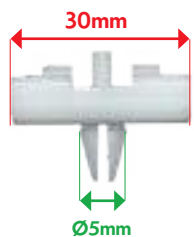
VB12036 AGRAFE VITRAGE R50, R52 et R53
