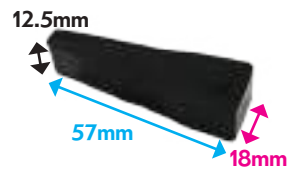
VB4000701 CALE ÉPAISSEUR Omega A (86-93)
