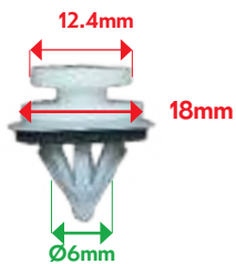
VB93305 AGRAFE MOULURE PB C4 Picasso
