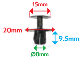
VB4000704 AGRAFE TOLE AUVENT
