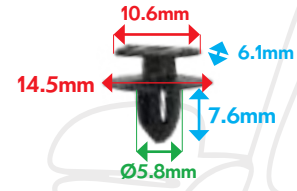
VB4000714 AGRAFE TOLE AUVENT
