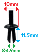
VB4000709 AGRAFE CACHE MOTEUR
