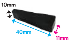
VB4000701 CALE CAOUTCHOUC 100/A6 (91-97)
