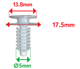
VB59405 AGRAFE PANNEAU DE PORTE modèles variés
