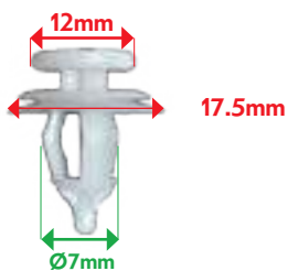
VB72205 AGRAFE PANNEAU PORTE Berlingo, Picasso et Saxo
