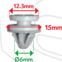
VB18255 AGRAFE PANNEAU DE PORTE Clio I, Megane, Trafic
