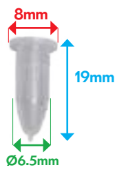
VB89427 TETINE DE PANNEAU DE PORTE AX, BX, Xantia, XM
